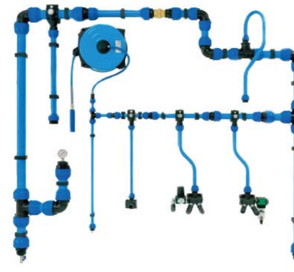
Rede de Ar Comprimido Easy-fit
